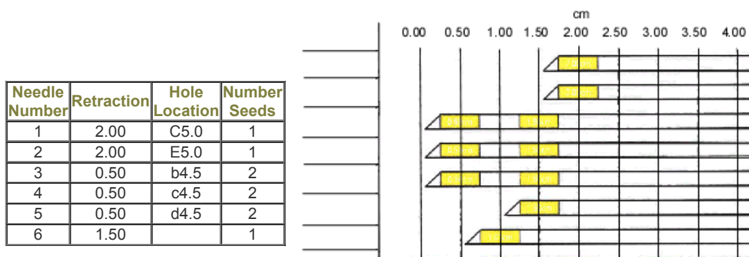
Fig 5 A la izquierda relación de las agujas, semillas y orificio. En la derecha, esquema de semillas dentro de agujas.
